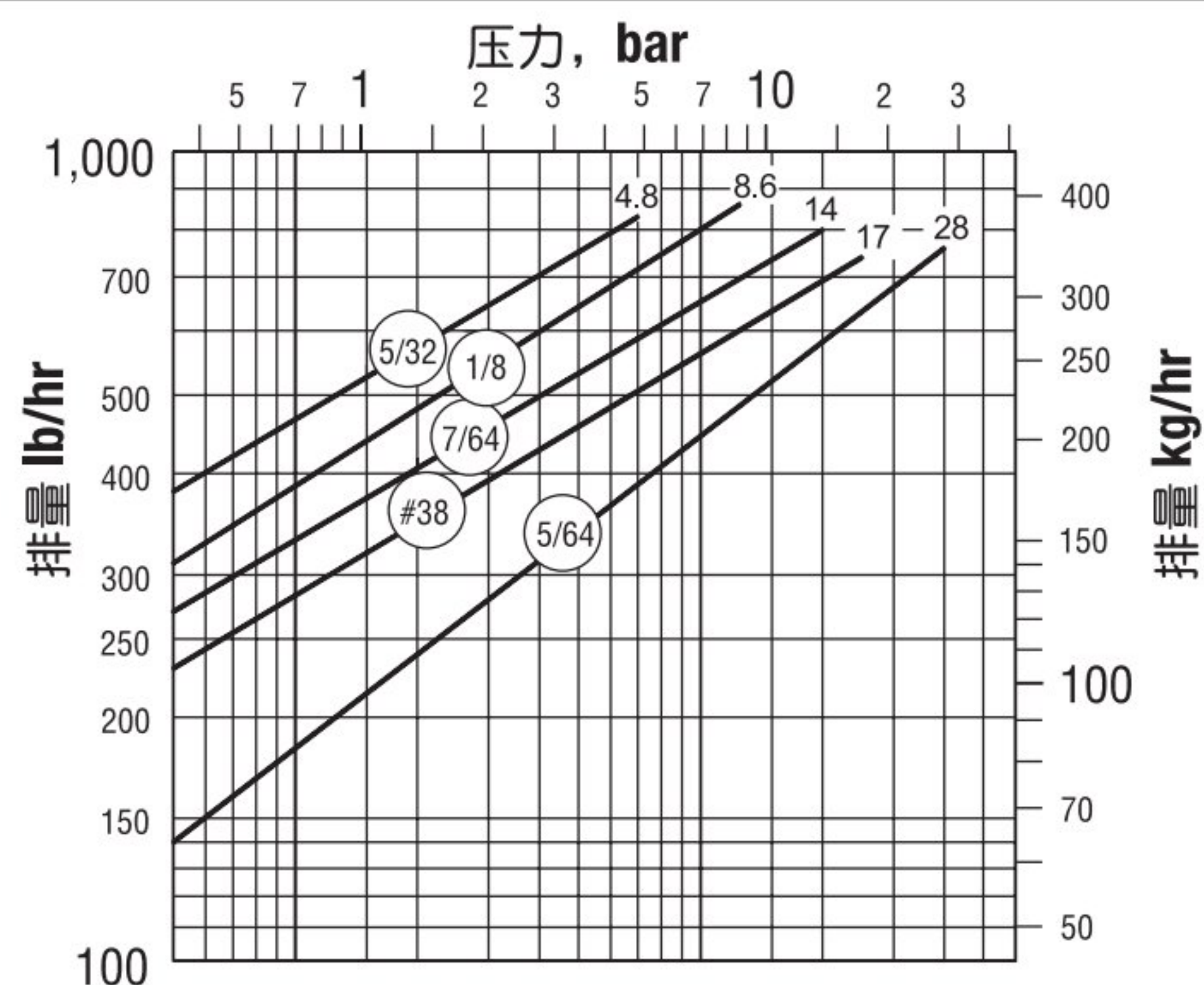
IB4011 型排量
