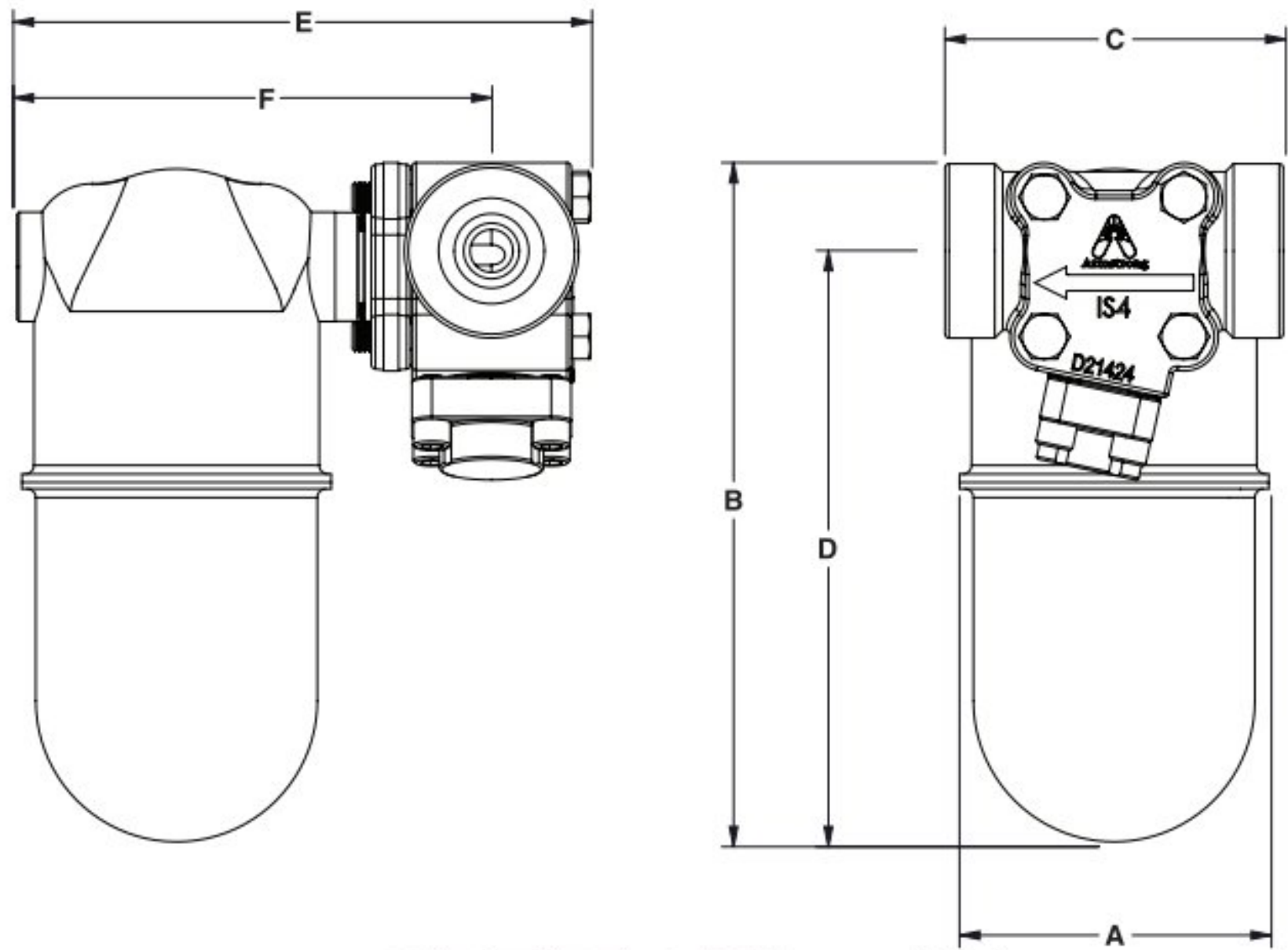
IB4022 型倒置桶疏水阀带 IS-4 接头
