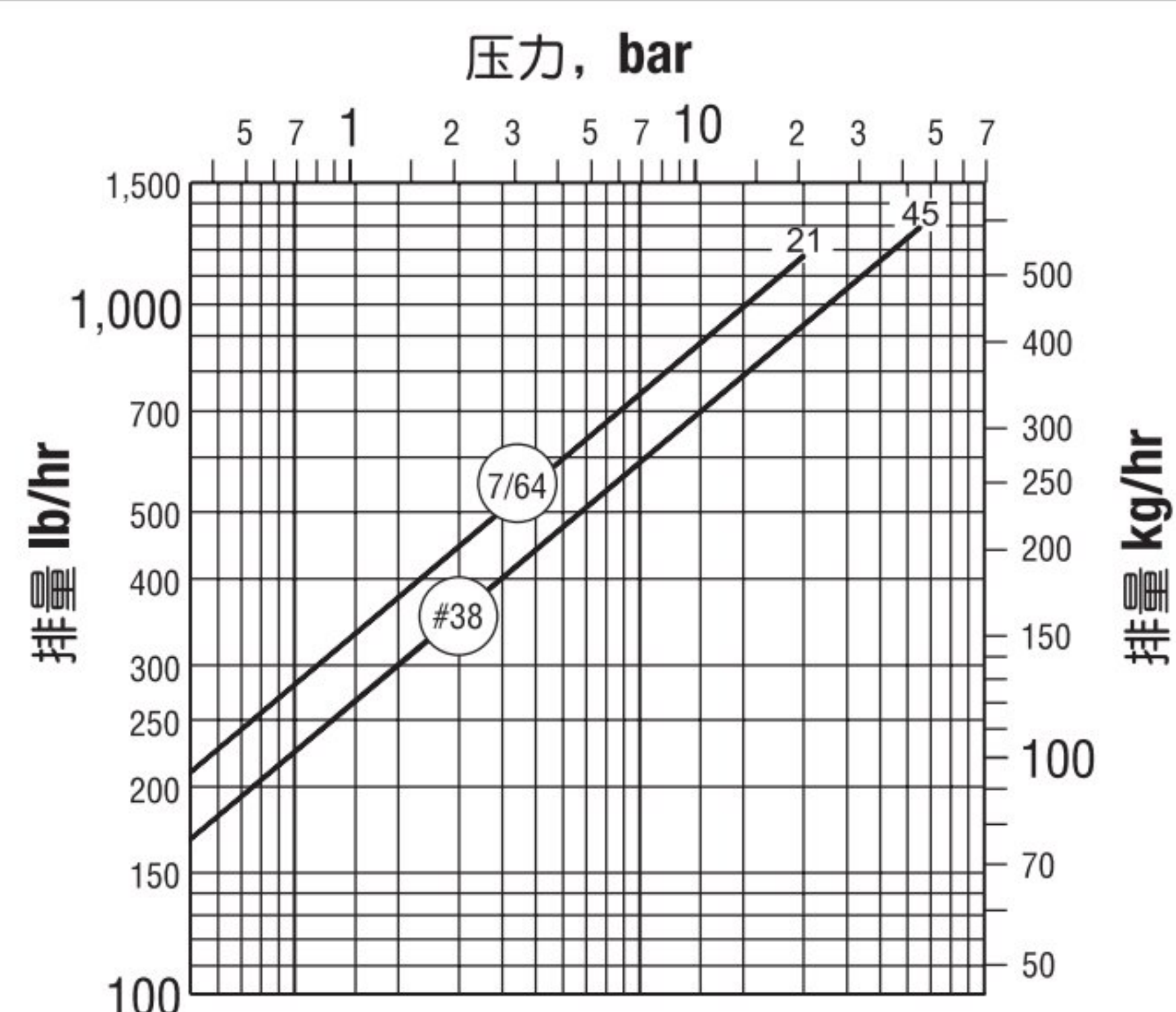
IB4022 型排量
